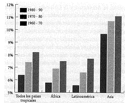
Gráfico 3 Tasa de deforestación tropical estimada (1960-1990)
