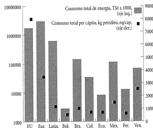
Gráfico 16 Consumo de energía (1997)
