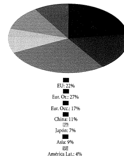
Gráfico 14 Emisiones mundiales de CO 2 (1995)
