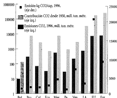
Gráfico 13 Emisiones de CO 2
